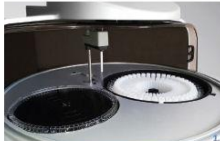
1. Optical carousel and sample/reagent tray Carosello ottico e piatto campioni/reagenti
